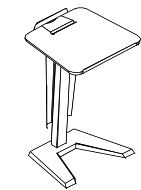
演讲台 Rostrum W580*D520*H1100
