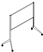
移动白板 Moveable White Board W1300*D690*H1850
