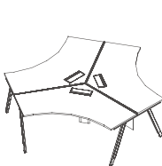
DN50 W2344*D2710*H750(mm)
