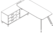
DN87L/R W1800*D1630*H750(mm) W2000*D1630*H750(mm)
