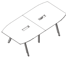
DN72 W2800*D1400*H750(mm) W3200*D1400*H750(mm) W3600*D1400*H750(mm)
