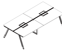
DN53 W2400*D1228*H750(mm) W2800*D1428*H750(mm) W3000*D1428*H750(mm) W3200*D1428*H750(mm)
