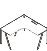
DN62L/R W1428*D1428*H750(mm) W1528*D1528*H750(mm) W1628*D1628*H750(mm)
