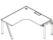
DN62AL/R W1428*D1428*H750(mm) W1528*D1528*H750(mm) W1628*D1628*H750(mm)
