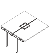
DN61A W1200*D1228*H750(mm) W1400*D1428*H750(mm) W1500*D1428*H750(mm) W1600*D1428*H750(mm)
