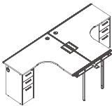
DN63A W1428*D2828*H750(mm) W1528*D3028*H750(mm) W1628*D3228*H750(mm)
