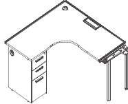
DN62BL/R W1456*D1428*H750(mm) W1556*D1528*H750(mm) W1656*D1628*H750(mm)
