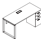
单人职员位主桌 DL60-2.CG W1200*D600*H750 W1400*D700*H750 W1500*D700*H750 W1600*D700*H750
