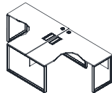
两人 L 工作位主桌 DL62-2.GJ W1400*D2812*H750 W1500*D3012*H750 W1600*D3212*H750
