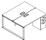
两人职员位主桌 DL61-2.CG W1200*D1212*H750 W1400*D1412*H750 W1500*D1412*H750 W1600*D1412*H750
