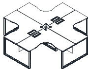
四人 L 工作位主桌 DL63-2.GJ W2812*D2812*H750 W3012*D3012*H750 W3212*D3212*H750
