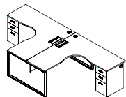
两人 L 工作位主桌 DL62-2.CG W1400*D2812*H750 W1500*D3012*H750 W1600*D3212*H750
